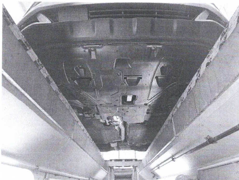
Bild 6 : Unterboden-Antriebsaggregat
